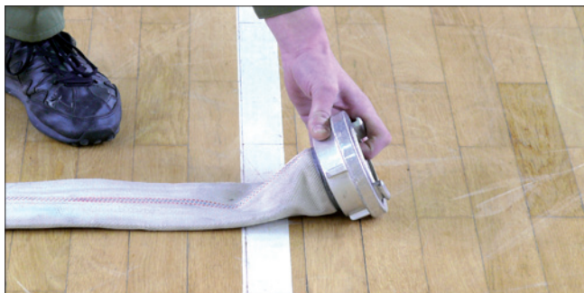
Abb. 43: Richtiges Ablegen der Kupplung des zweiten B-Schlauches.
